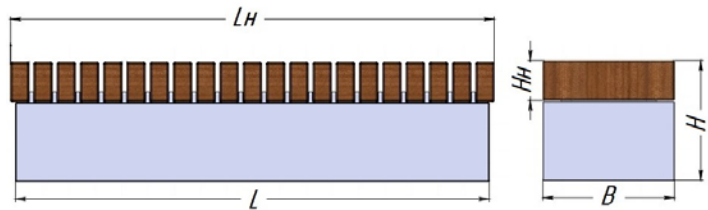
Блок бетон
